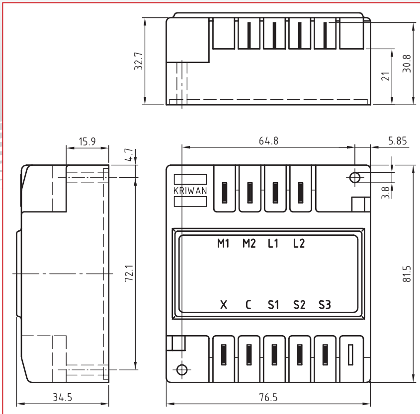
«« DIMENSION PRINT
