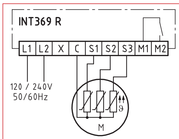
«« CONNECTION DIAGRAM
